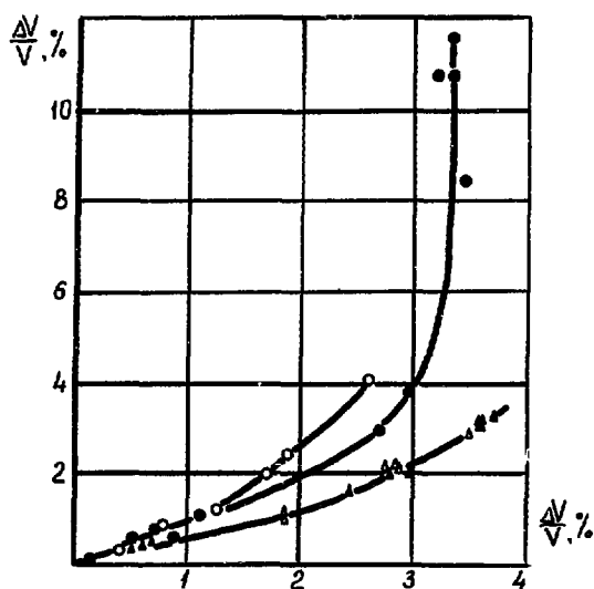
Рис.2. Расширение кристаллических решеток графита (o) и карбида кремния (Δ) в зависимости от расширения алмаза.
