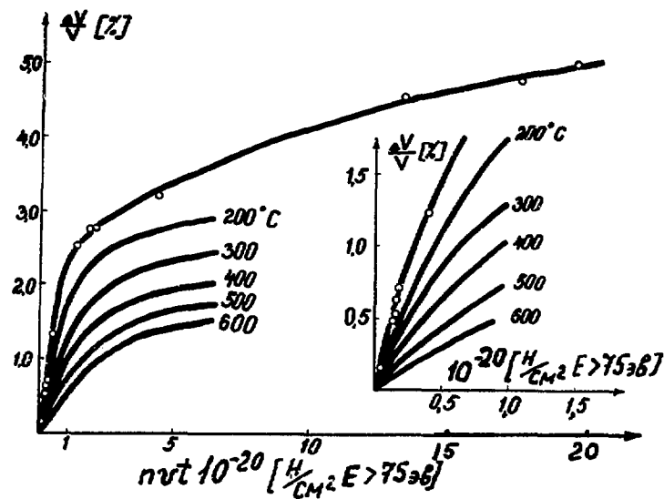
Рис.1. Изменение объемного расширения кристаллической решетки алмаза от температуры и дозы нейтронного облучения (рабочий канал реактора РЭТ).
